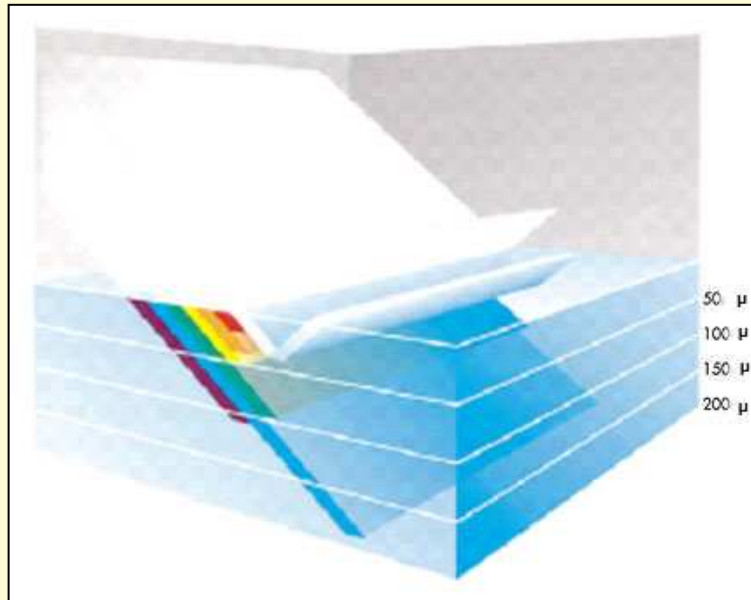
Εικόνα 15: Ανάμεσα στο 3 και 30 τοις εκατό του φωτός του ηλίου αντανακλάται στην επιφάνεια της θάλασσας. Έπειτα σχεδόν τα επτά χρώματα του πρίσματος φωτός απορροφούνται το ένα μετά το άλλο στα πρώτα 200 μέτρα, εκτός του μπλε φωτός (Ωκεανοί, Έλντερ και Περνέττα, σελ. 27)
