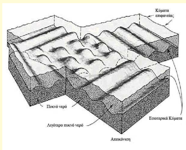
Εικόνα 16: Εσωτερικά κύματα σε διεπιφάνεια ανάμεσα σε δυο στρώματα νερού διαφορετικών πυκνοτήτων. Το ένα είναι πυκνό (το χαμηλό), το άλλο είναι λιγότερο πυκνό (το ανώτερο). (Ωκεανογραφία, Γκρός, σελ. 204.)
