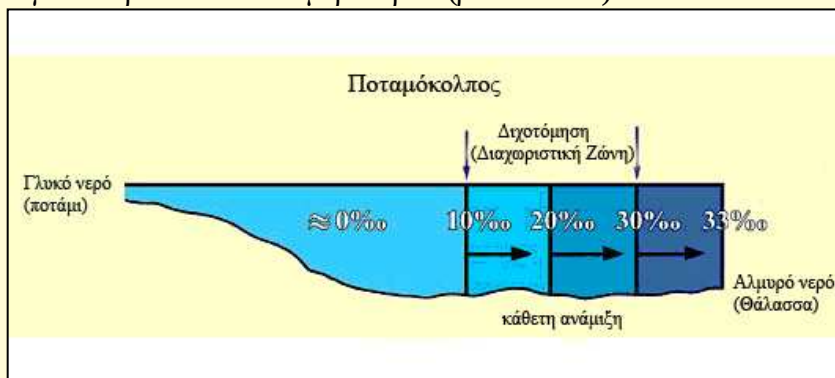
Εικόνα 14: Διαμήκης τμήμα που δείχνει αλμυρότητα (τοίς χιλίοις ‰) σε ένα ποταμόκολπο. Βλέπουμε εδώ τη διχοτόμηση (ζώνη του διαχωρισμού) ανάμεσα στο γλυκό και το αλμυρό νερό. (Εισαγωγική Ωκεανογραφία, Θούρμαν, σελ. 301, με μια μικρή ενίσχυση).
