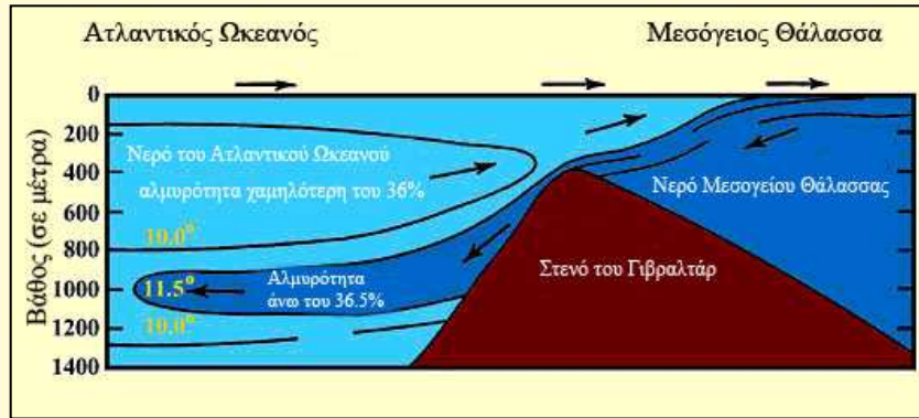
Εικόνα 13: Το νερό της Μεσογείου Θάλασσας, καθώς εισέρχεται στον Ατλαντικό από το Γιβραλτάρ με τα δικά του θερμά, αλμυρά, και λιγότερο πυκνά χαρακτηριστικά, εξ' απίας του εμποδίου που ξεχωρίζει ανάμεσά τους. Η θερμοκρασία είναι σε βαθμούς Κελσίου (C). (Θαλάσσια Γεωλογία, Κουένεν, σελ. 43, με μια μικρή ενίσχυση.)
