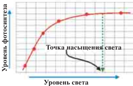
Кривая фотосинтеза под воздействием света
